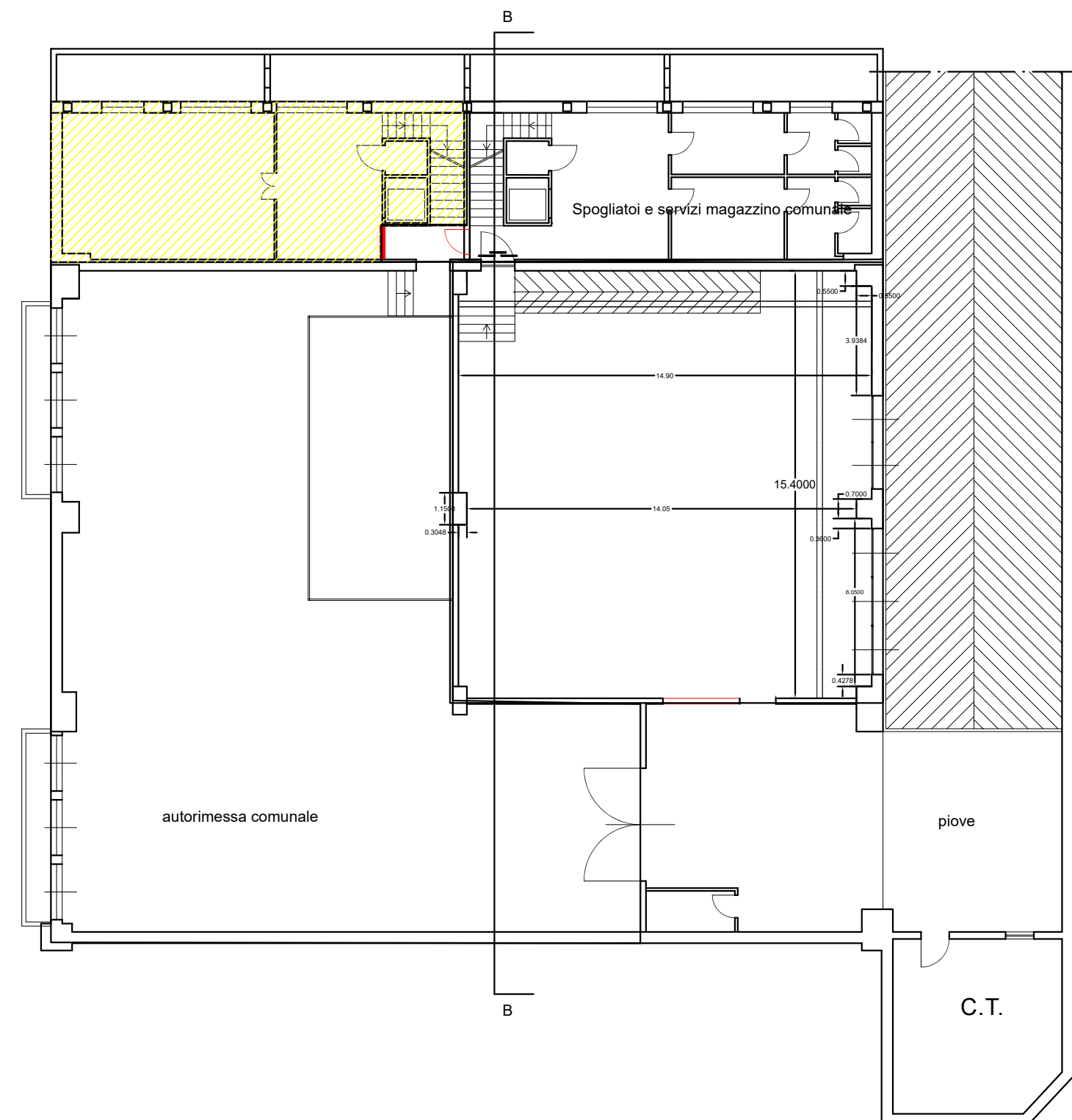
Pianta Piano Interrato
